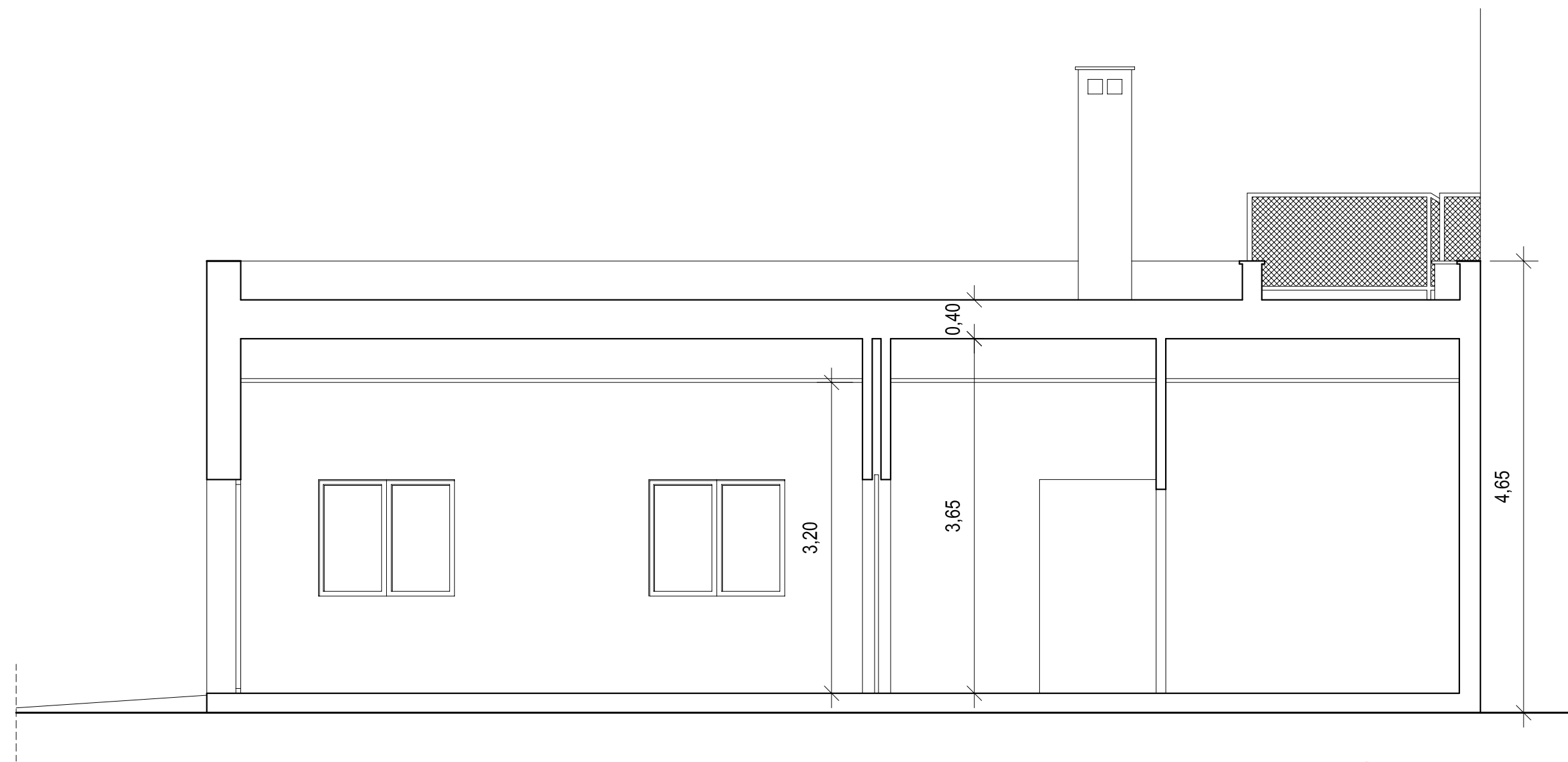
SECCIÓN A-A'
