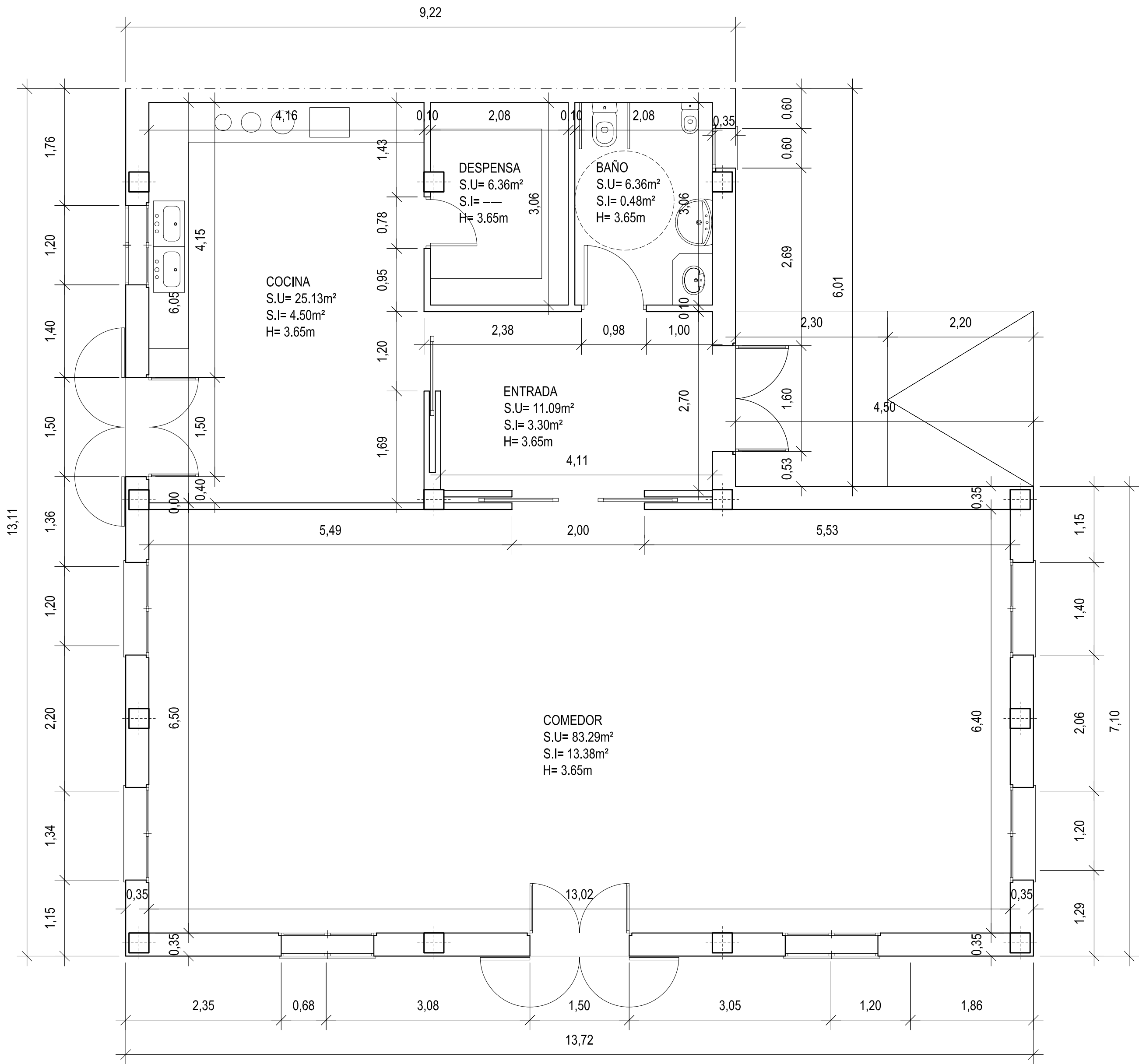
PLANTA CONSTRUCTIVA
